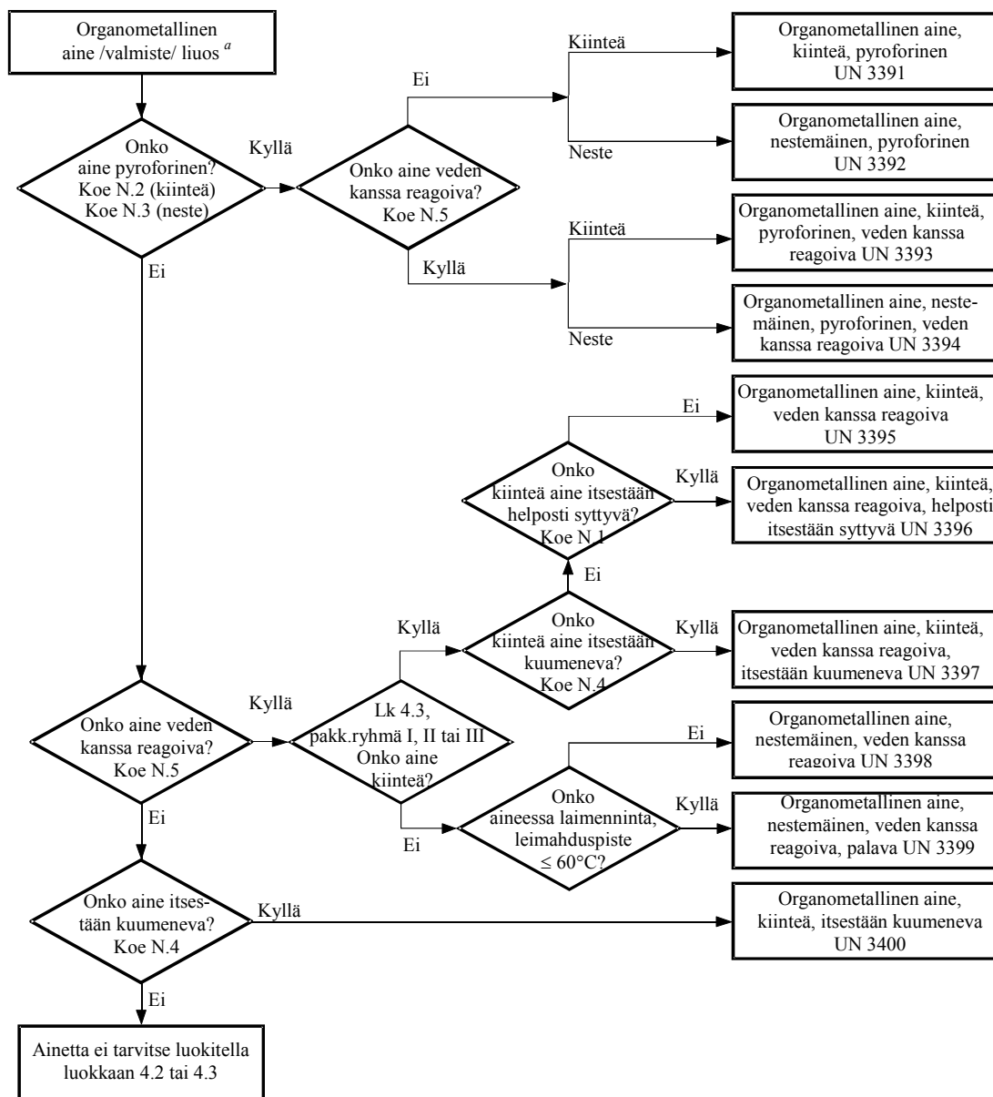
Kuva 2.3.5: Vuokaavio organometallisten aineiden luokittelumiseksi luokkiin 4.2 ja 4.3 b
