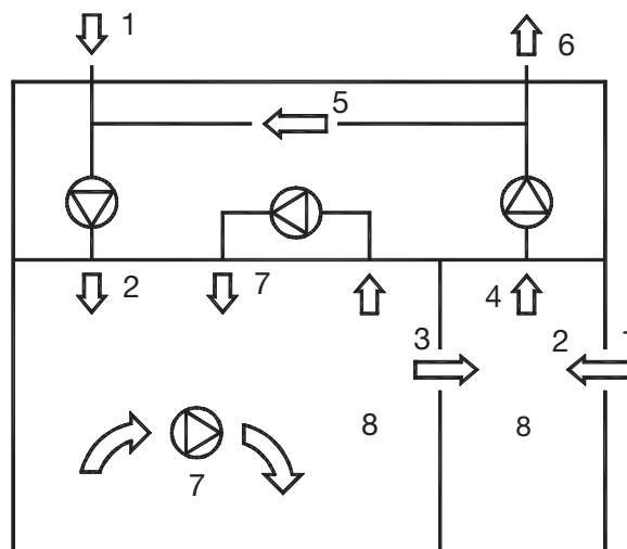
Figur 1. Benämningar på luftströmmar: 1. Ute-luft, 2. Tilluft, 3. Överluft, 4. Frånluft, 5. Återluft, 6. Avluft, 7. Cirkulationsluft, 8. Inneluft.
