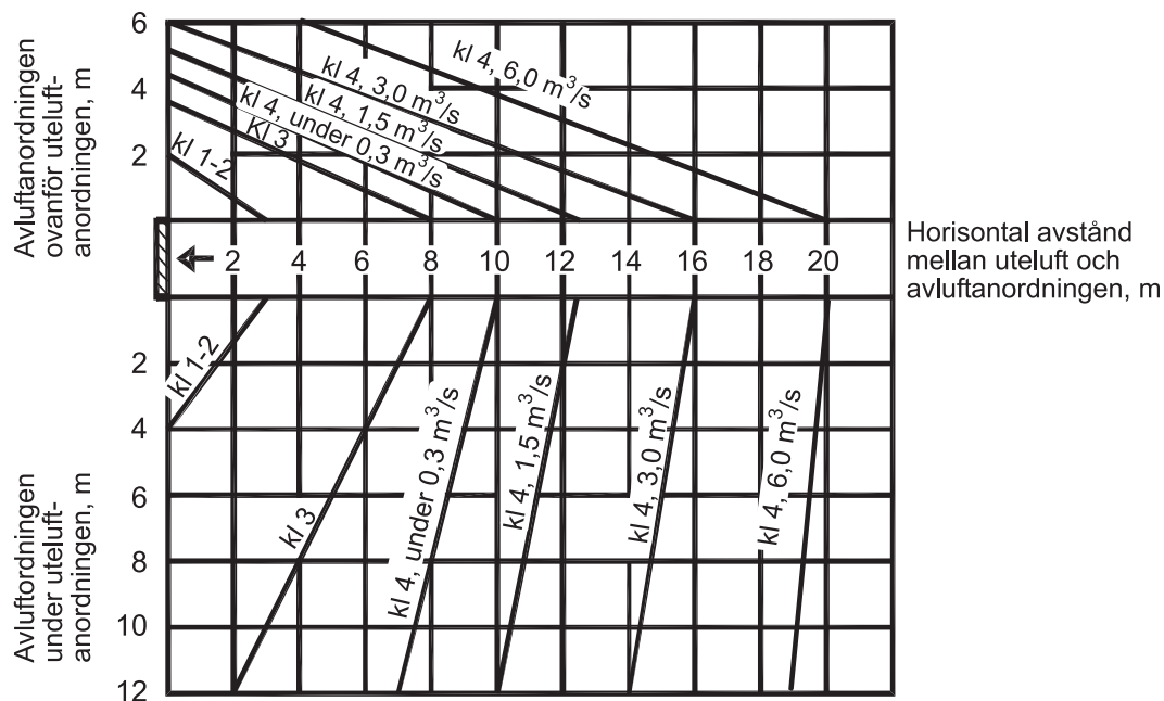
Figur 2. Avstånd mellan avluft- och uteluftsöppningar. Värden mellan linjerna kan uppskattas.
