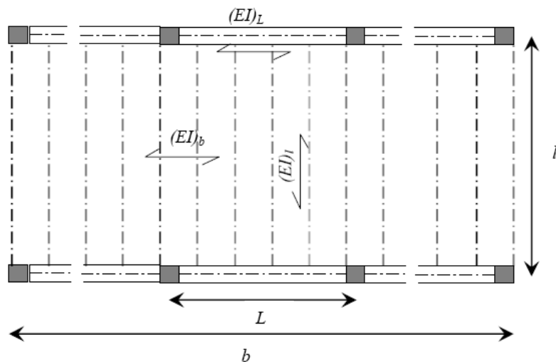
Bild 1. Ett typiskt delområde av ett mellanbjälklag som omfattar ytplattan, golvbalkar och huvudbalkar.
