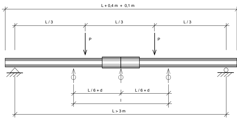
Bild 1. Böjprov på skarvad påle
