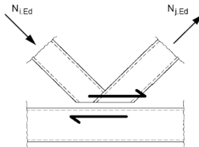
Bild 1. Överlappsförband. Livstängernas skärning på ramstången.
