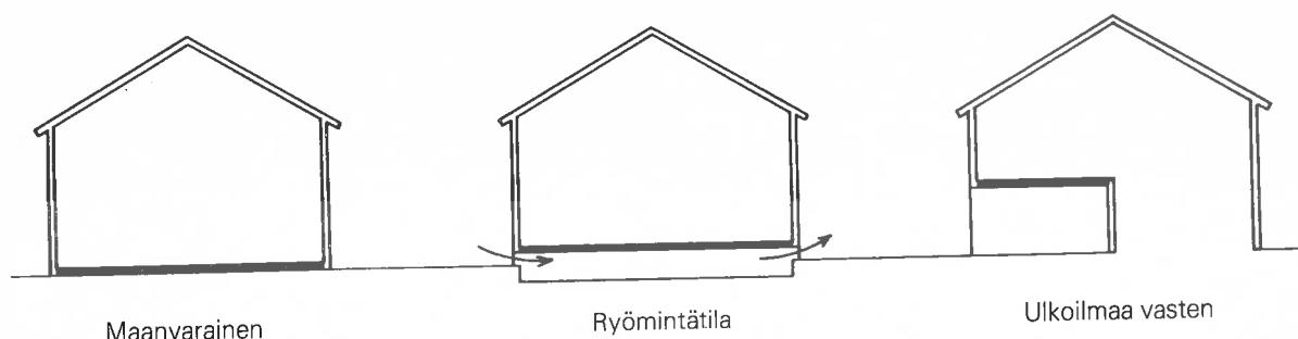
Kuva 2. Alapohjan erilaisia rakennetyyppejä
