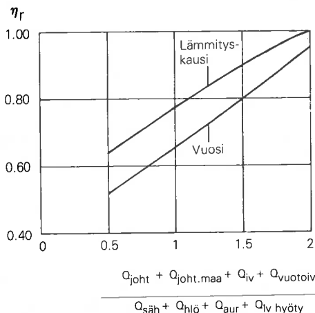
Kuva 4. Ideaalinen sisäisten energioiden hyväksikäyttöaste \eta_r
