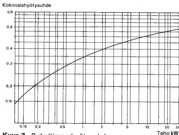
Kuva 7 Puhaltimen hyötysuhde
