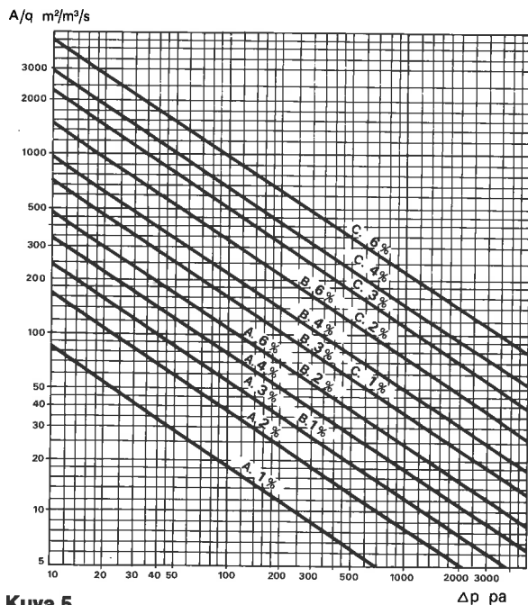
Kuva 5 Kanavistojen tiiviysluokan valintakäyrästä
