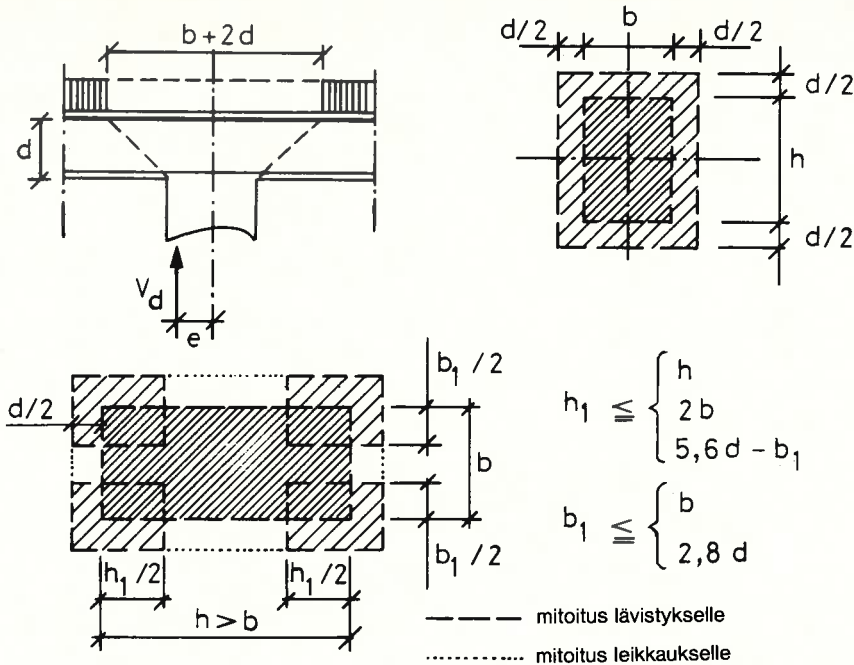
Kuva 2.15 Laatan lävistys
