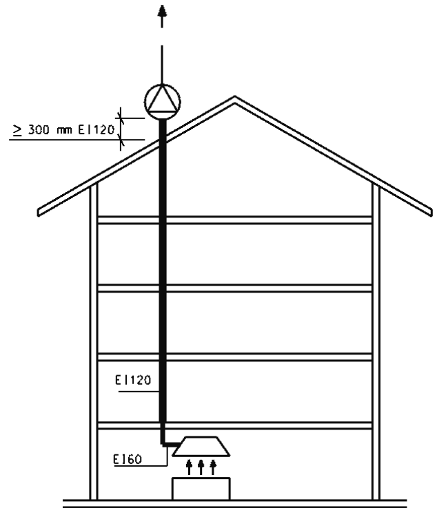
Kuva 1. Esimerkiksi ammattimaisesti käytetyn keittiön kohde- poistokanavan palonkestävyys.
