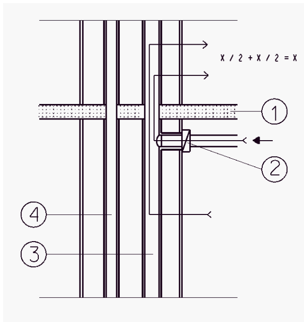
Kuva 5. Roilon palonkestävyys.
