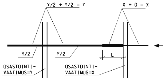
Kuva 4. Palo-osaston läpi siihen avautumatta kulkevan kanavan palonkestävyys, kun ei käytetä palonrajoittimia. Kuvas- sa esitetty paksunnettua paloeristystä edellyttävä pituus L valitaan taulukosta 1.
