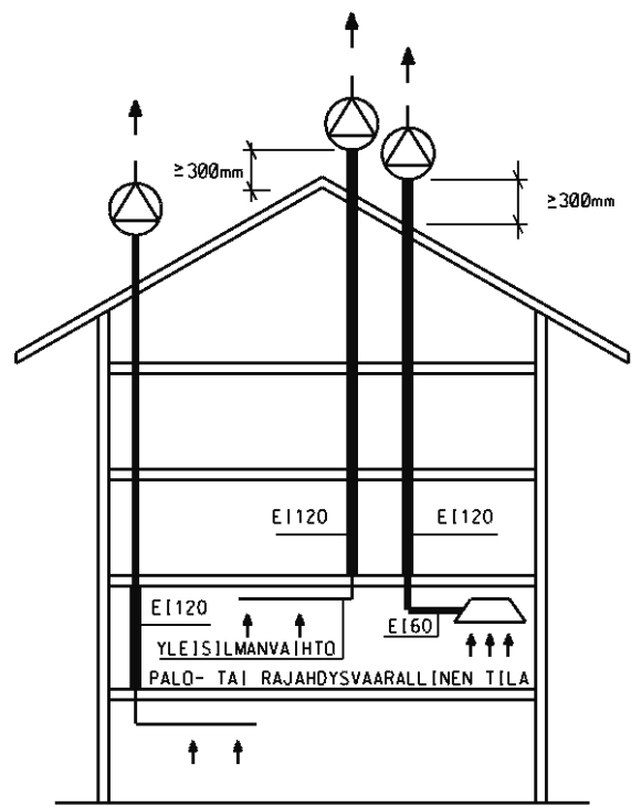
Kuva 2. Palo- tai räjähdysvaarallisen tilan ilmakanavien palon- kestävyys.
